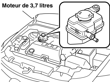
Moteur de 3,7 litres
